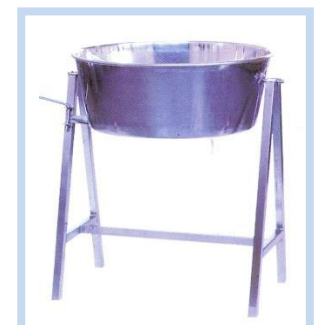
TINAS PARA LA CASEIFICACIÓN DE PASTA HILADA FRESCA (MOZZARELLA)
